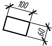
поз. 18 (М1:10) t6x100x60 С245
