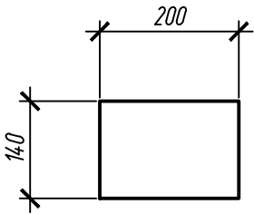
поз. 19 (М1:10) t10x200x140 С245
