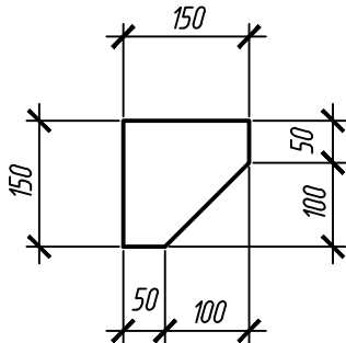
поз. 23 (М1:10) t10x150x150 С245
