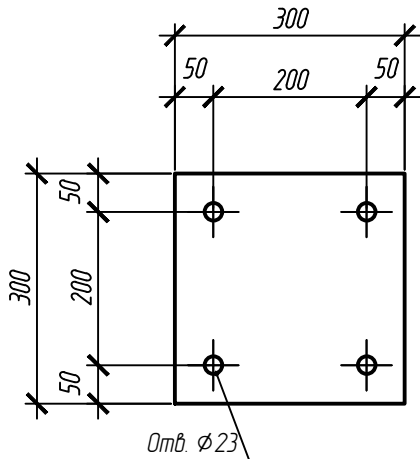
поз. 20 (М1:10) t10x300x300 С245
