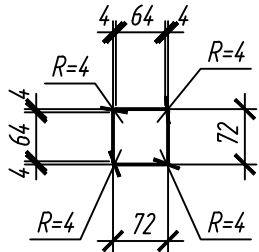
поз. 21 (М1:10) t3x72x72 С245
